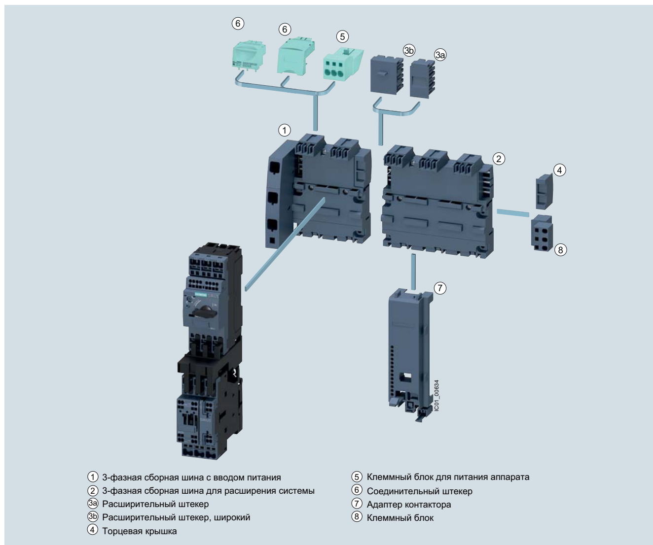
Система электропитания SIRIUS 3RV29
