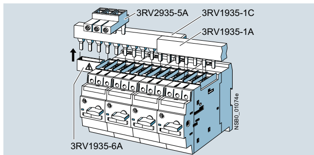
Системы 3-фазных шин SIRIUS, типоразмер S2
